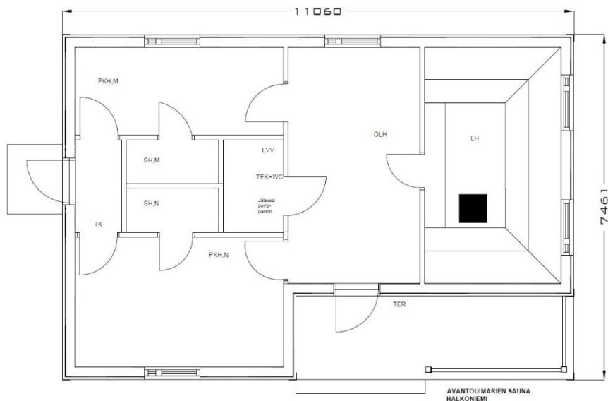
Pohjapiirustus ennen laajennusta.
