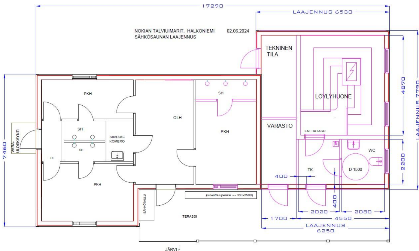
Laajennus lisätty pohjapiirustukseen.
